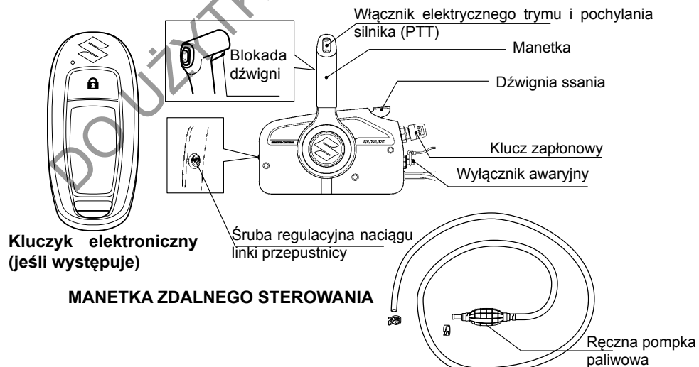
PRZEWÓD PALIWOWY
